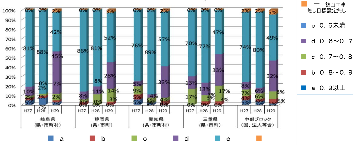
施工時期等の平準化(平準化率(稼働金額 \beta ))
