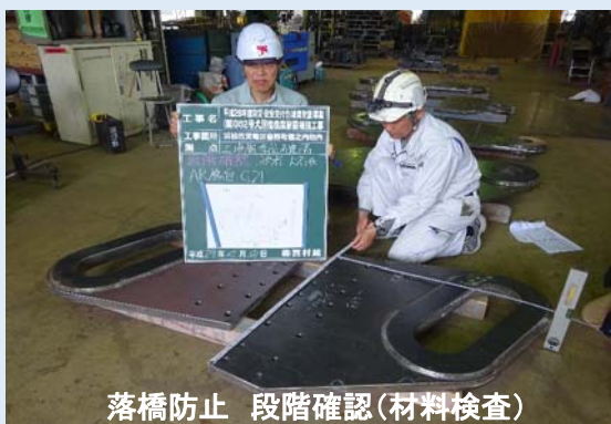
落橋防止 段階確認(配筋検査)
