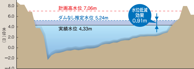
浦川地点の河川横断面図
