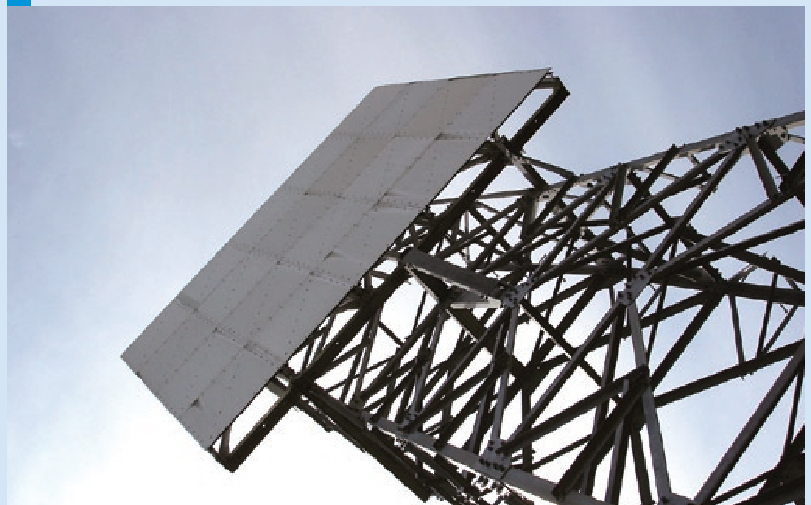
山間にある雨量観測所や水位観測所などの施設とダムとの間の無線通信のために、電波を反射させる施設。
