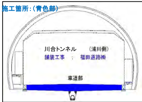
計画図
