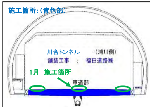
計画図
