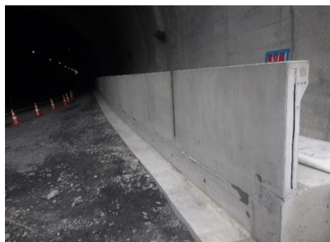
監査路壁完成
