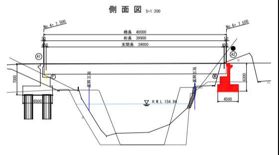
橋台工側面図
