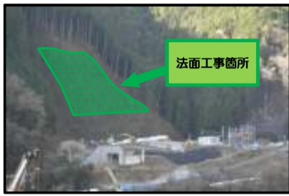
現場全景 大千瀬川対岸より撮影
