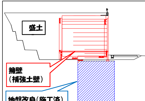
擁壁施工方法 (コンクリートの板を積上げ盛土をします。)
