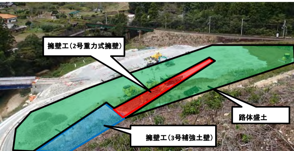
工事箇所
