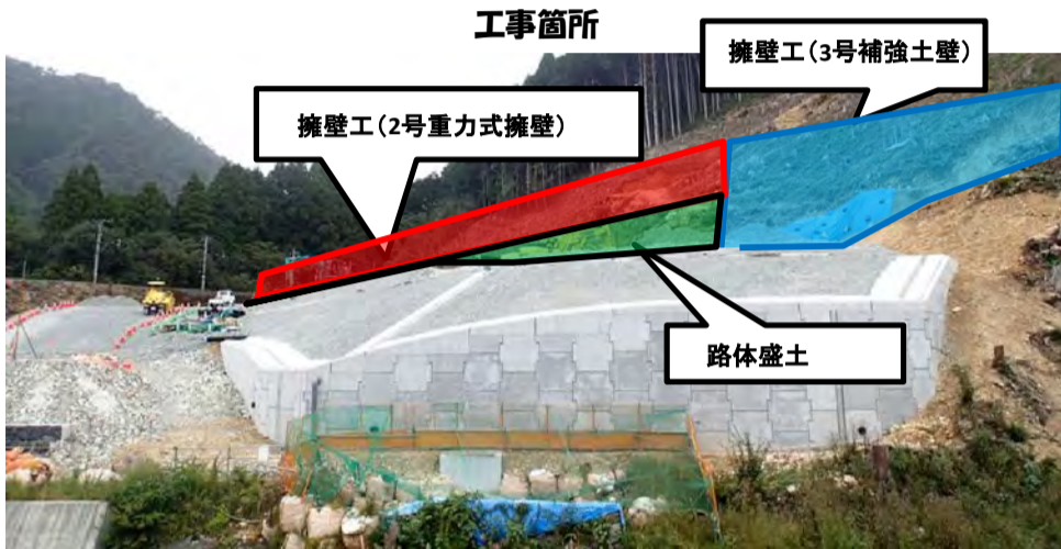
工事箇所
