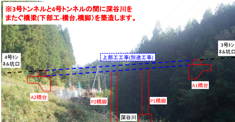
施工箇所 (西側から撮影)
