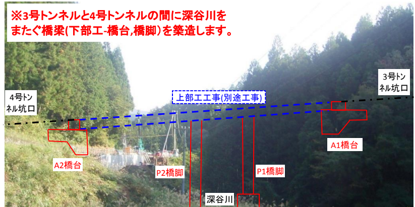
施工箇所 (西側から撮影)
