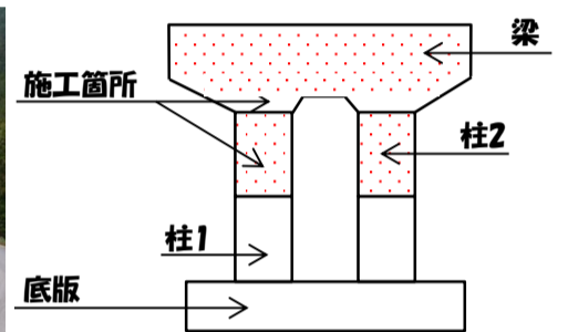
橋脚図面
