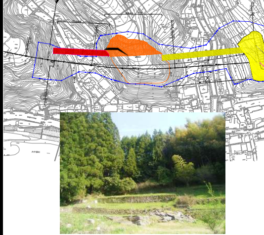
本線土工(仮橋)部
