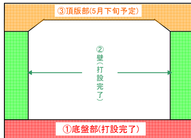
函渠工コンクリート打設順序と施工時期
