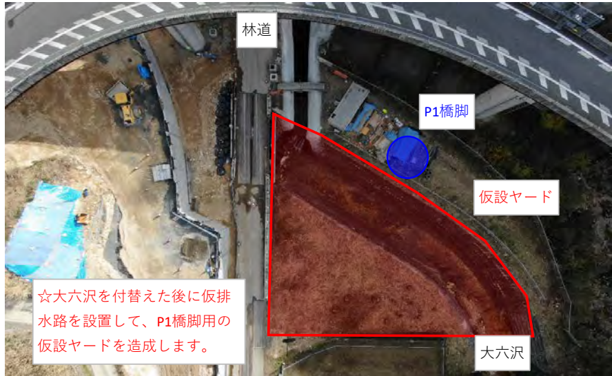
9号橋P1橋脚の仮設ヤード造成工事
