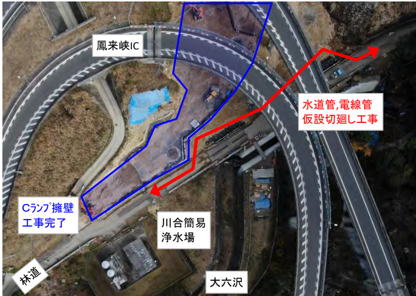
用地外の落石対策工事
