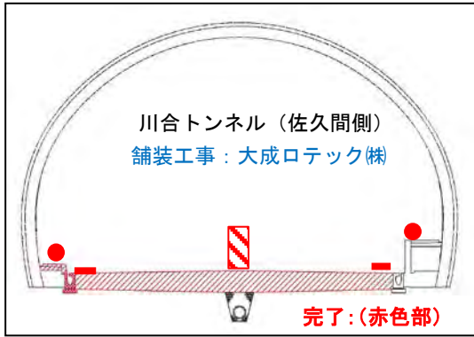
完成予想図(川合側坑口)
