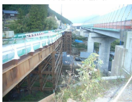
川合2号橋仮橋進捗状況
