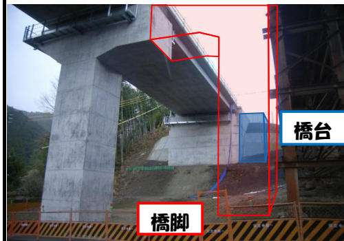
2号橋 橋台・橋脚
