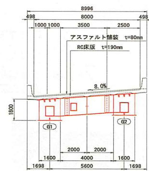
断面図 S=1:100
