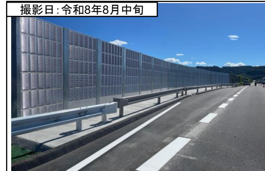
⑦大代IC下り線(非常駐車帯新設)
