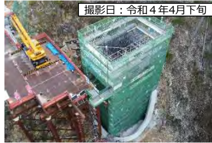
②8号橋 (仮称) P2橋脚
