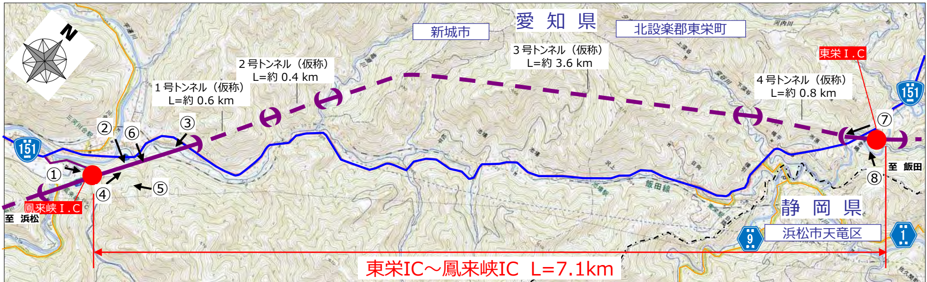
③7号橋(仮称)
