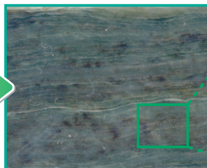
石英
