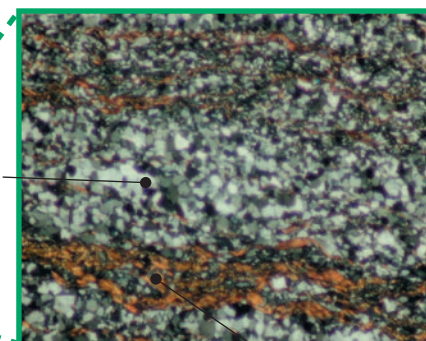
ガーネット
