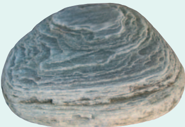
結晶片岩
