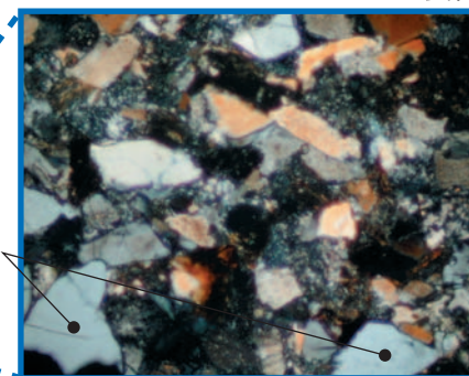
長石
