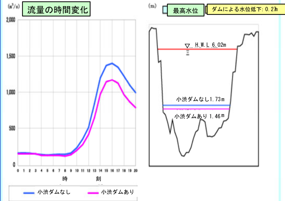
宮ヶ瀬地点の流量と水位
