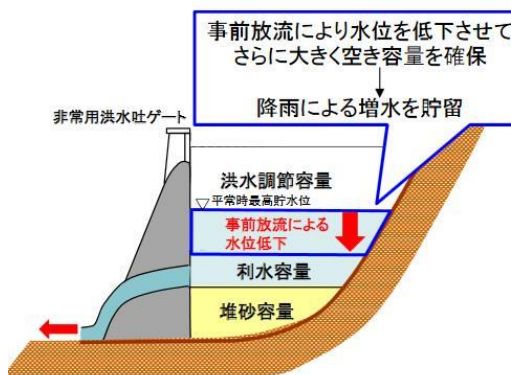
多目的ダムの事前放流イメージ
