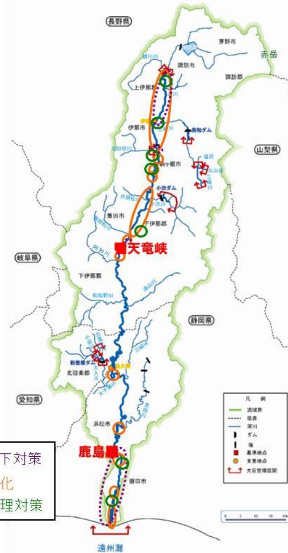
河川整備計画に基づく整備位置図
