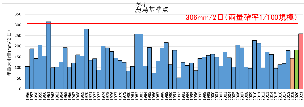
基準点における年最大雨量(mm/2日)の整理
