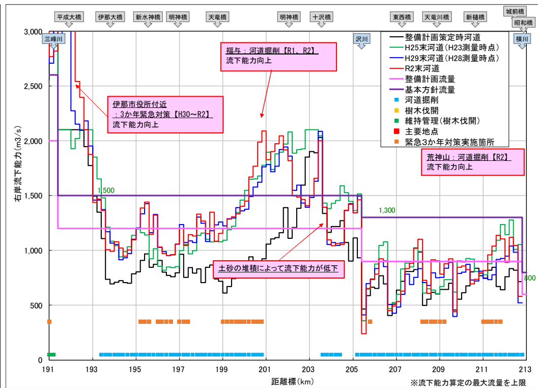
流下能力_HWL評価(伊那・伊北地区)
