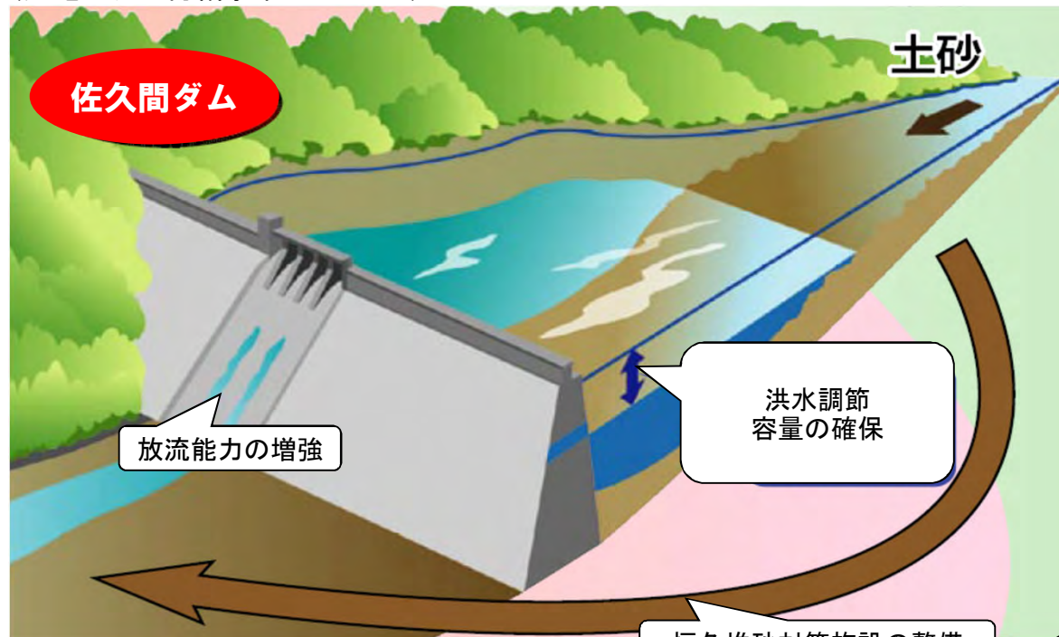
〈天竜川ダム再編事業のイメージ〉
