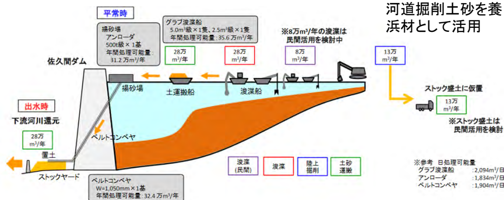
佐久間ダムにおける恒久堆砂対策のイメージ
