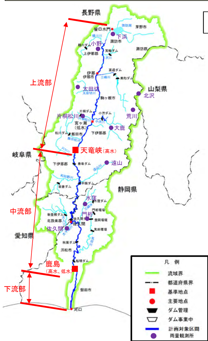
■レーダー雨量(令和2年7月出水)
