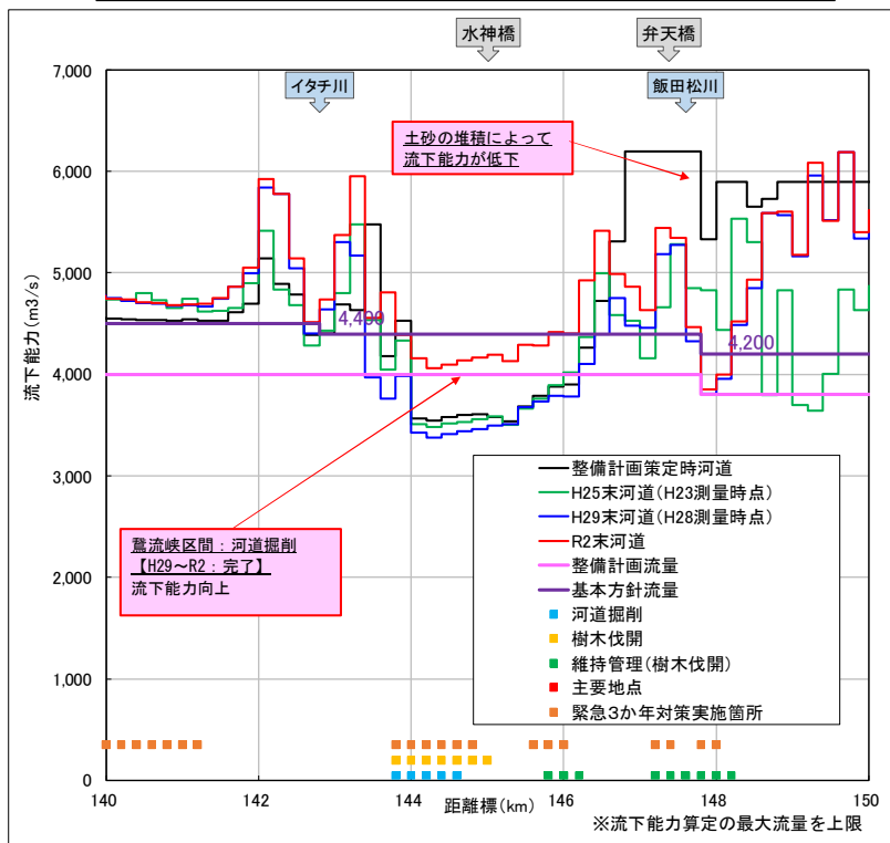
流下能力_HWL評価(鷺流峡区間)
