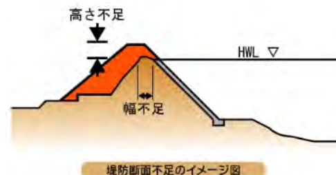
堤防断面不足のイメージ図
