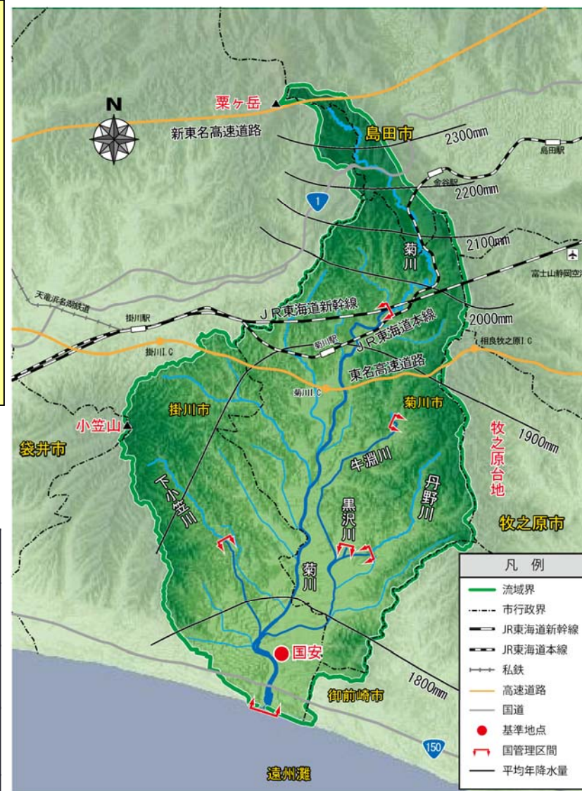
流域図及び平均年降水量分布図
