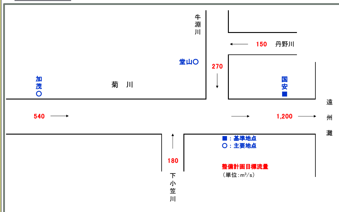
流量配分図
