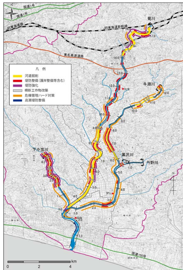
概ね30年間の主な整備位置図
