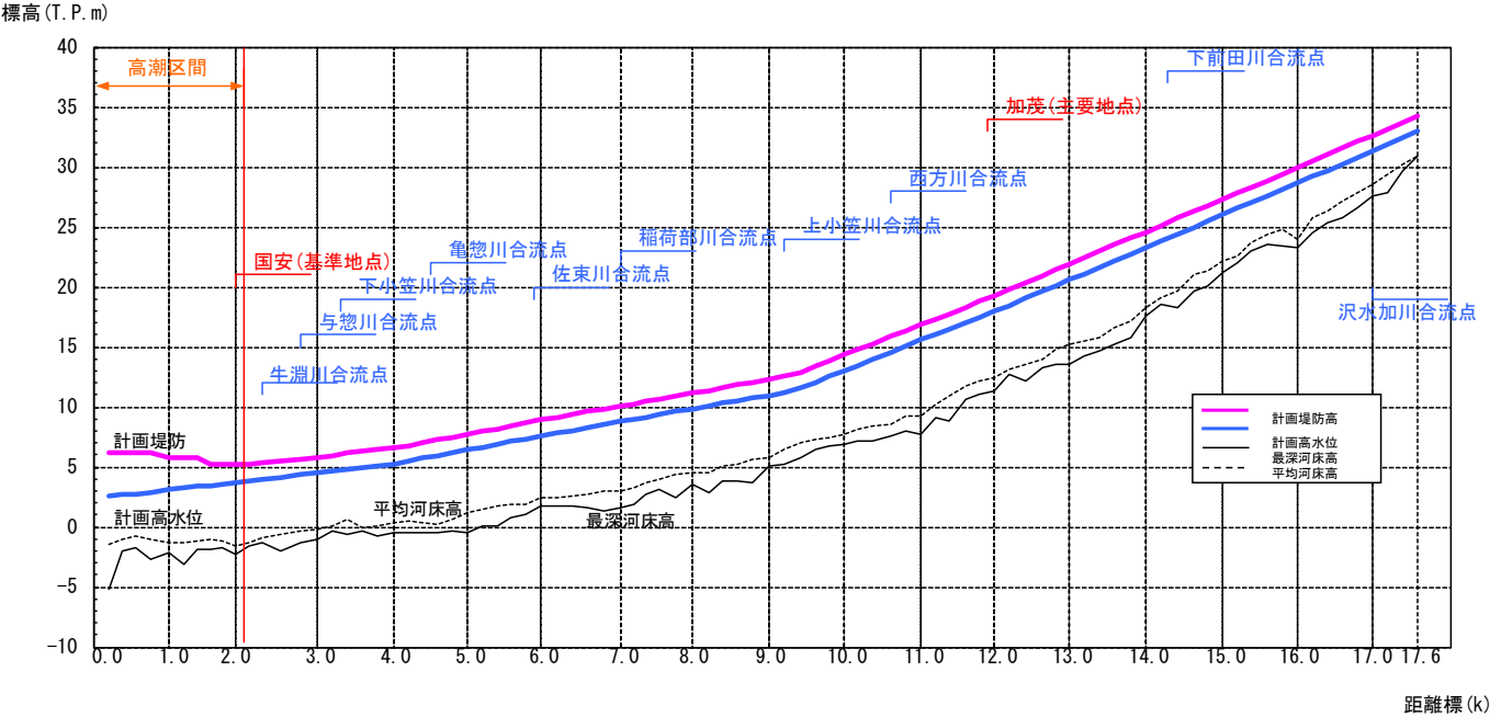
菊川本川計画縦断面図 (0.0~17.6km)
