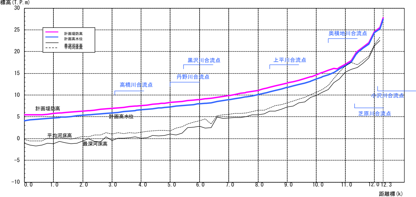
牛淵川計画縦断面図 (0.0~12.3km)
