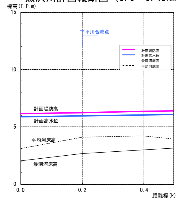
黒沢川計画縦断面図 (0.0～0.45km)
