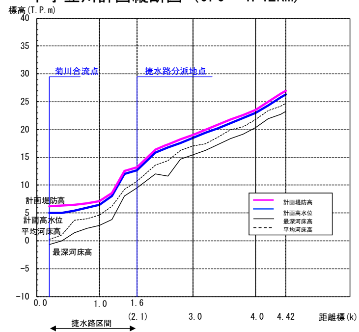
下小笠川計画縦断図 (0.0~4.42km)
