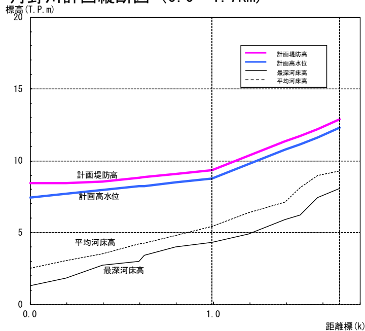
丹野川計画縦断面図 (0.0～1.7km)
