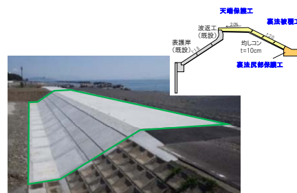
緊急対策のイメージ (粘り強い構造の海岸堤防)
