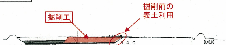
横断図
