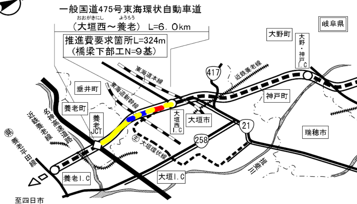
平面図
