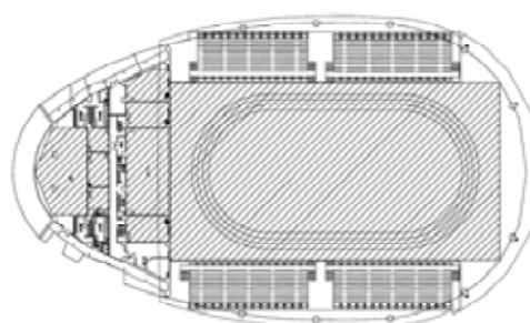
多目的ドーム内の平面図
