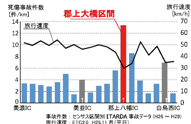
図1 国道156号（美濃IC付近～白鳥西IC付近）延長あたりの死傷事故件数 および 旅行速度
