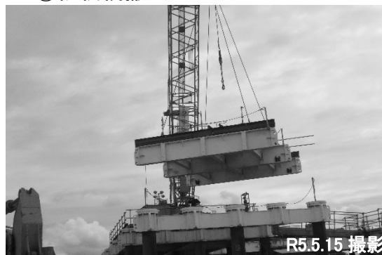
▼⑤仮栈橋撤去
