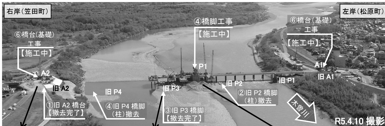
▼⑥A2 橋台基礎
