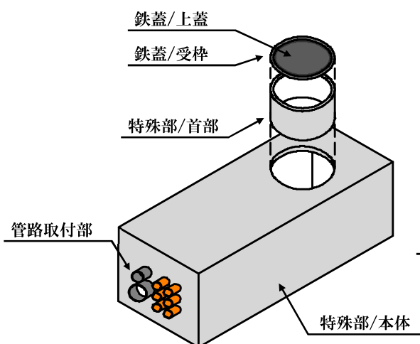
図 3-1 特定した弱点部(特殊部)
