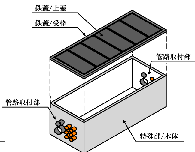
図 3-1 特定した弱点部(特殊部)
