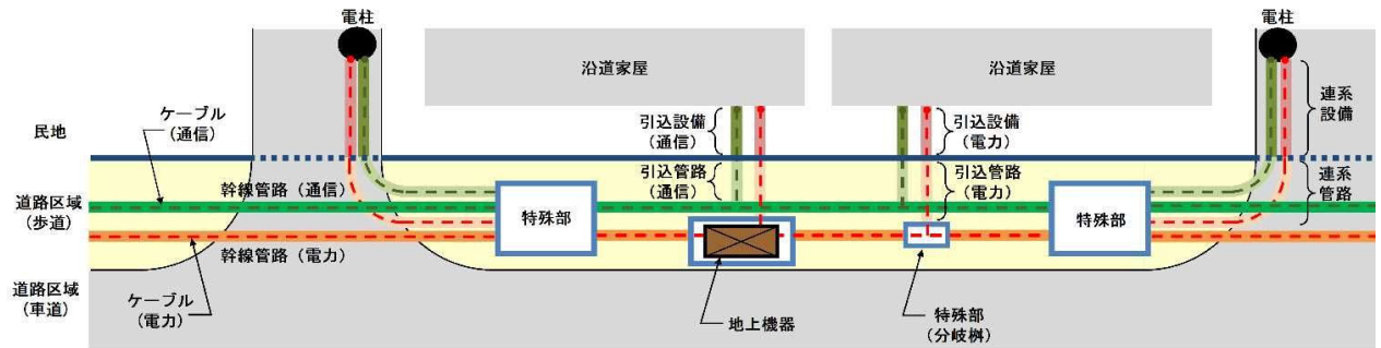
図 1-2 構造と管理区分
