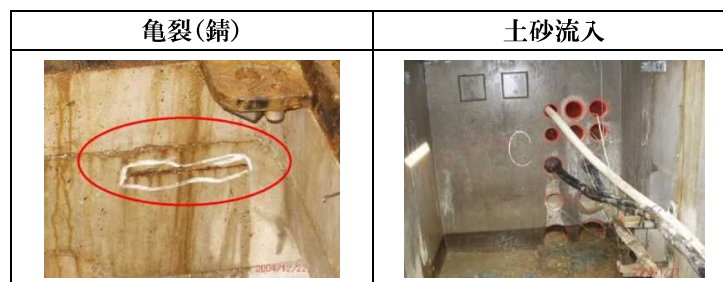
図 3-3 特殊部(本体・首部)の損傷例
