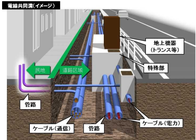
図 1-1 電線共同溝施設
