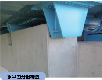
水平力分担構造
