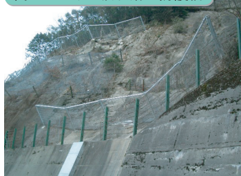
高エネルギー吸収落石防護柵
