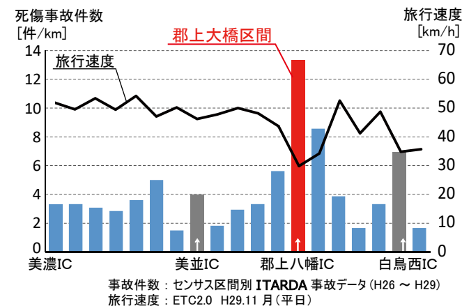
図1 国道156号（美濃IC付近～白鳥西IC付近）延長あたりの死傷事故件数 および 旅行速度
