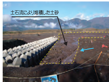
土石流発生後 第7上流床固工 堆積状況
