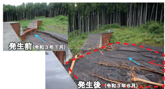
風祭川第1砂防えん堤工
