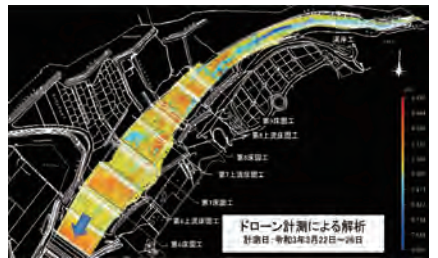
UAV写真による堆砂量解析
