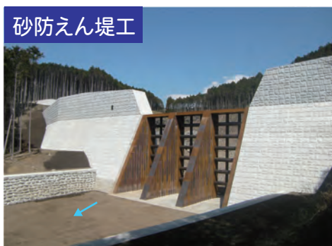
千束第5砂防えん堤工
