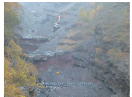
溪床対策工（2号横工） ヘリコプターによる無人化施工状況
