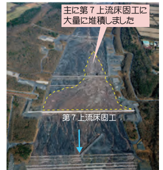
土石流発生後 大沢川遊砂地工 堆積状況
