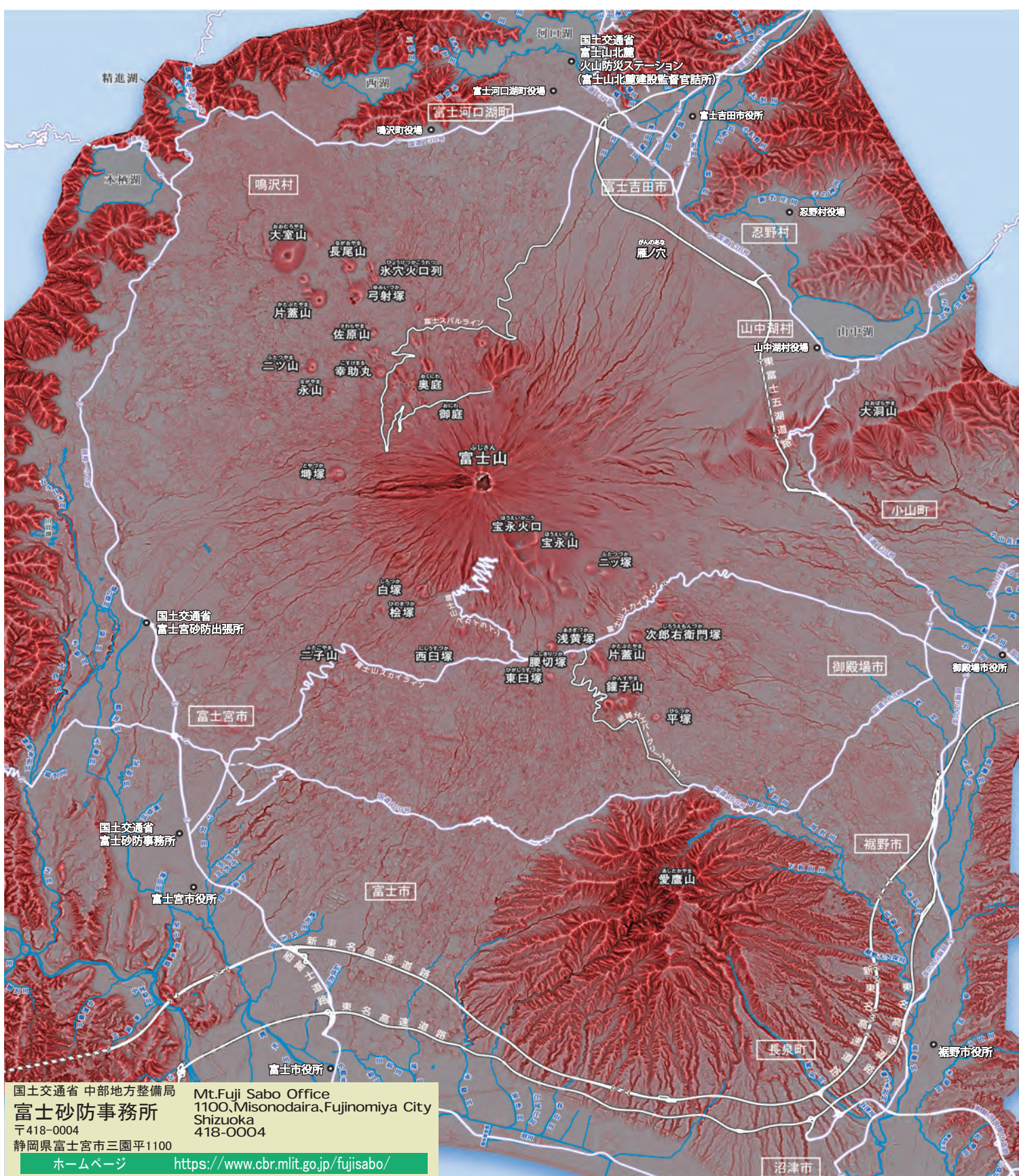
赤色立体図
