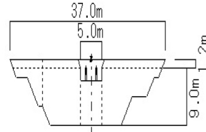
副堰堤正面図
