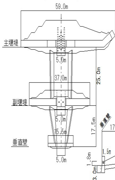
平面図
