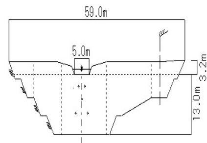
副堰堤正面図
