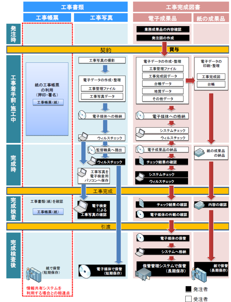
図 土木工事における電子納品・電子検査の流れ (紙で工事帳票を利用する場合)
