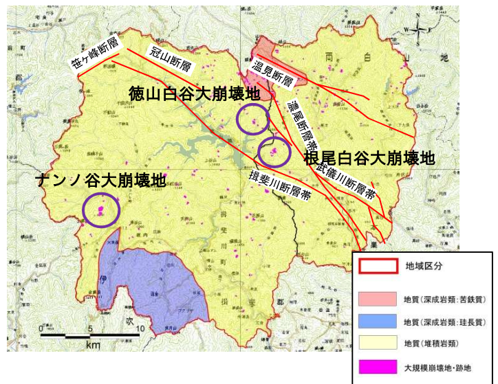
管内の活断層と過去の主な深層崩壊
