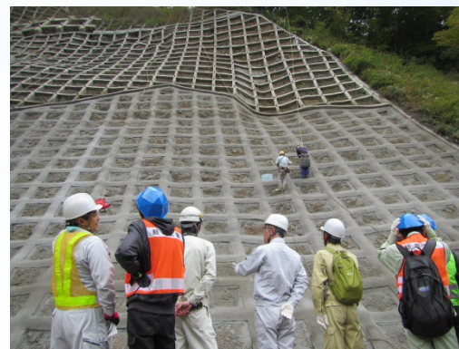
法面对策工の作業を見学 (八草山腹工事)
