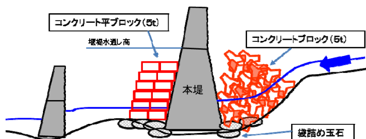
図1 応急対策工事イメージ
