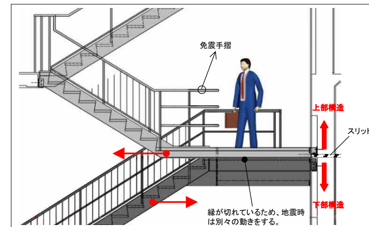
地下階段の免震構造
