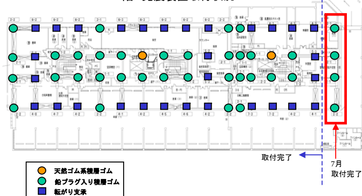
B1階 免震装置取付状況
