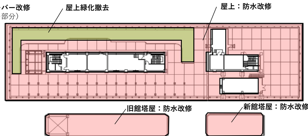
屋上・塔屋平面図
